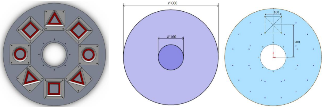
图 11 待装配体圆形铝板尺寸图
