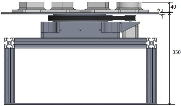
图 10 待装配体圆台侧视图（单位：mm）
